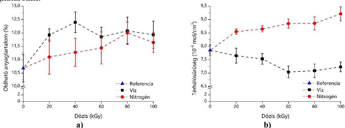
2. ábra A vizsgált gumiőrlete oldható anyagtartalma a); és térhálósűrűsége b)
