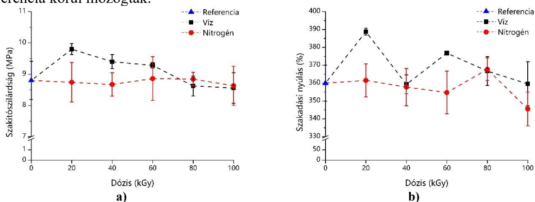
3. ábra A GTR tartalmú vulkanizátumok szakítószilárdsága a); és szakadási nyúlása b)
